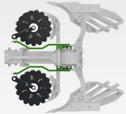
Coutre circulaire crénelé, Ø 600 mm, avec support long
